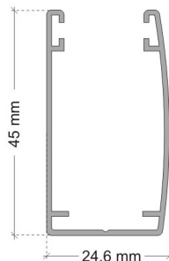
Coupe de la coulisse
