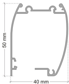
Coupe du boîtier
